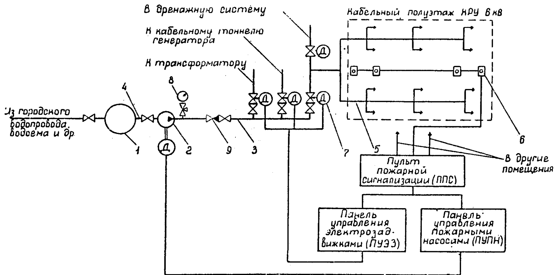
Принципиальная схема установки водяного пожаротушения:
